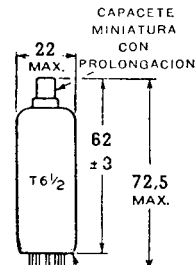
BOTON PEQUEÑA, MINIATURA, 9 PATITAS
