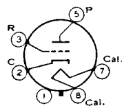
B: 12 SF5 SC: 12 SF5-GT
