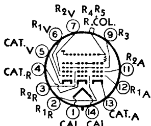
14AH ULTOR = R_4 + R_5 + COL. + R ELECTRODO DE ENFOQUE = R_3
