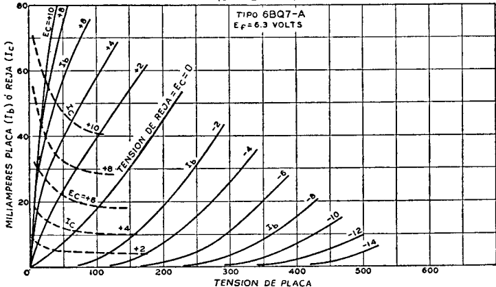
CARACTERÍSTICAS MEDIAS DE PLACA (CADA SECCION)
