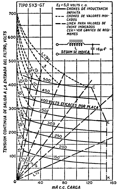
CARACTERISTICAS DE TRABAJO CIRCUITO DE ONDA COMPLETA CON CHOKE DE ENTRADA AL FILTRO
