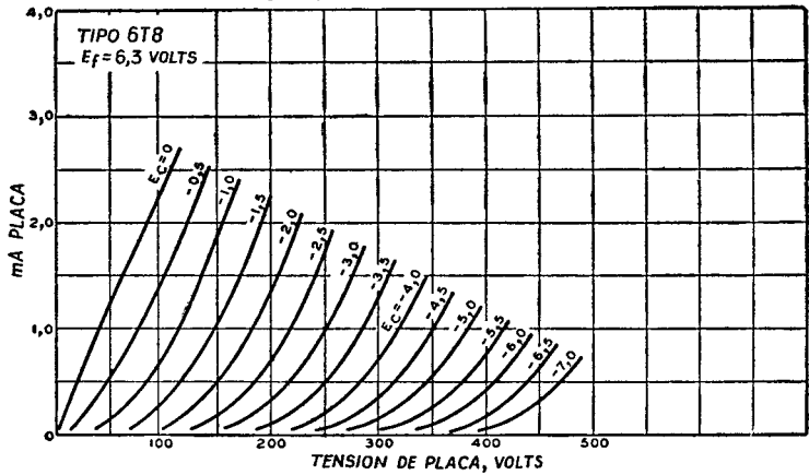
CARACTERISTICAS MEDIAS DE PLACA
