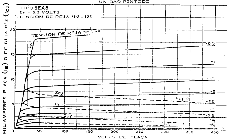
CARACTERÍSTICAS MEDIAS UNIDAD PENTODO
