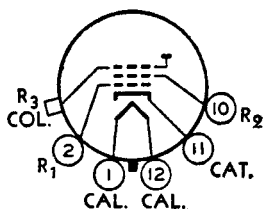
12D ULTOR = R_3 + COL.
