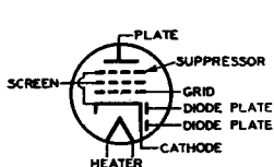
DUPLIX-DIODE PENTODE
