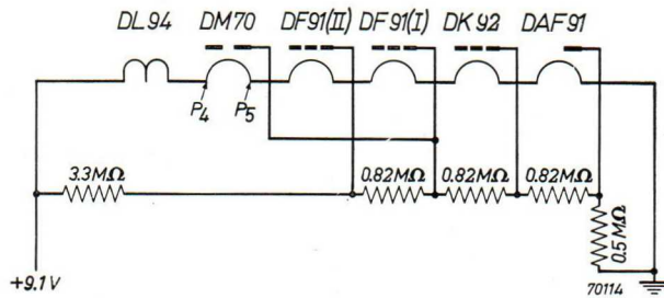
Fig. 113. The A.G.C. circuit.
